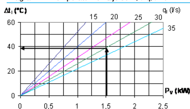
Diagram 2 – Temperatur forhøjelse P_v \rightarrow q_l \rightarrow \Delta t_l
